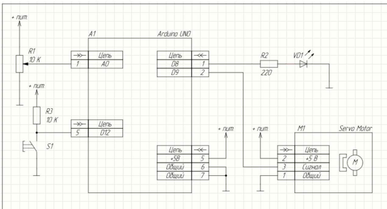
Рисунок. Электрическая принципиальная схема
